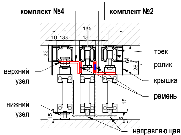
Вариант Б (фиксация ремня)
