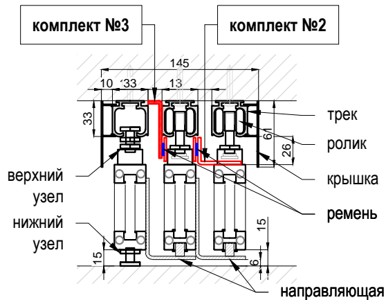
Вид сверху с закрытыми створками
