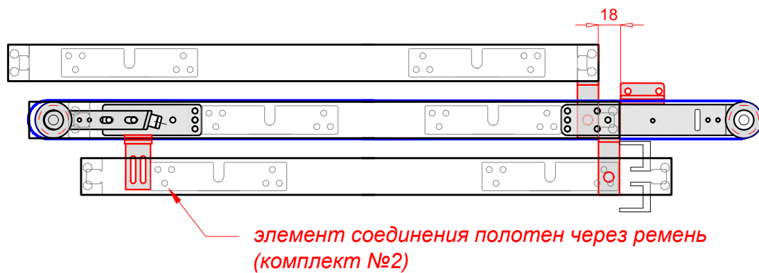
Вид сверху с открытыми створками
