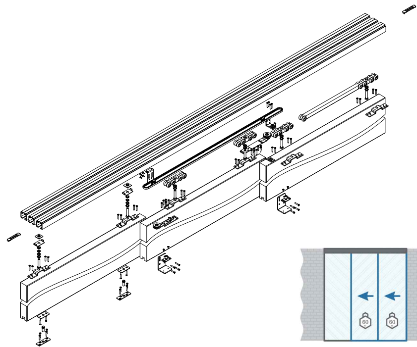
Верхний узел крепления неподвижной створки
