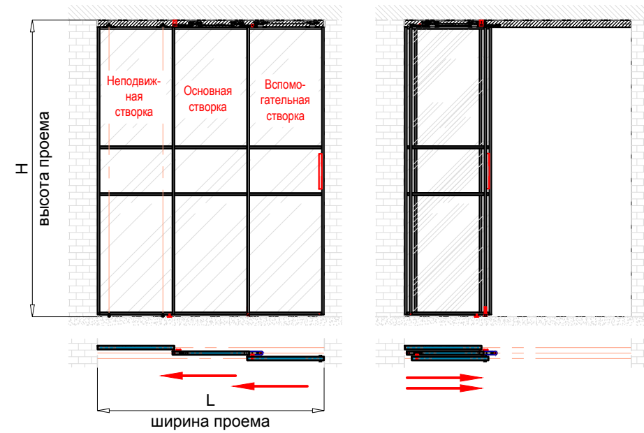
Вид прямо с закрытыми створками
