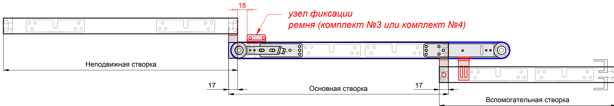
Вид сверху с открытыми створками
