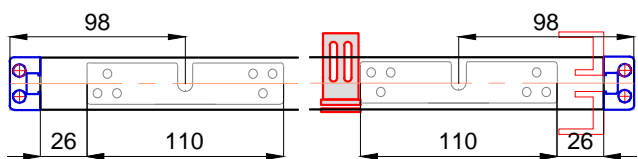
Створка (левая)
