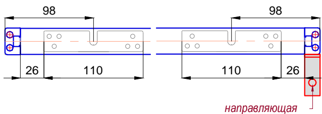
Створка (левая)
