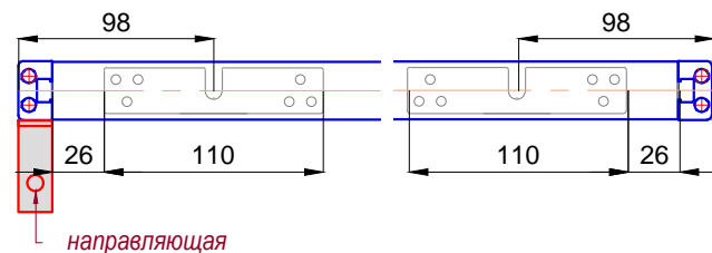
Створка (правая)
